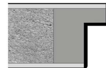
Bezspoinowe obrzeże: jednorodna powłoka obrzeża płyty drzwiowej
