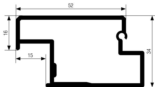
Listwa uchwytova metallic-line (aluminium/stal nierdzewna)
