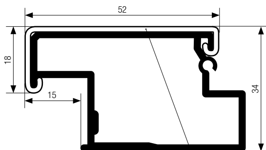
Listwa zamkowa nakładana (nakładka) color-line/decor-line Listwa zamkowa (element dolny) color-line/decor-line (aluminium)
