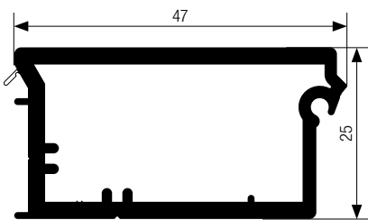
Listwa zamkowa acoustic-, decor- i color-line
