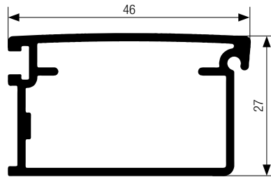
Listwa zamkowa metallic-line (aluminium/stal nierdzewna)
