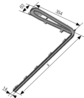
Prowadnica ślimakowa prawa i lewa: x=400 / 500 / 600 mm Pojemność 600 mm
