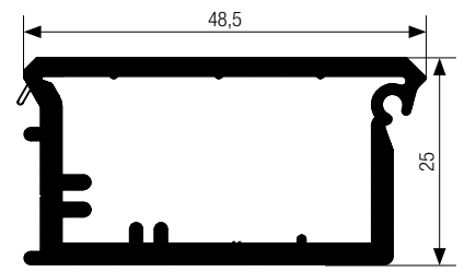
Flächenbündige Griffleiste Dekor für Rolladenprofil E9
