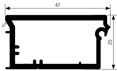
Griffleiste acoustic-, decor- und color-line
