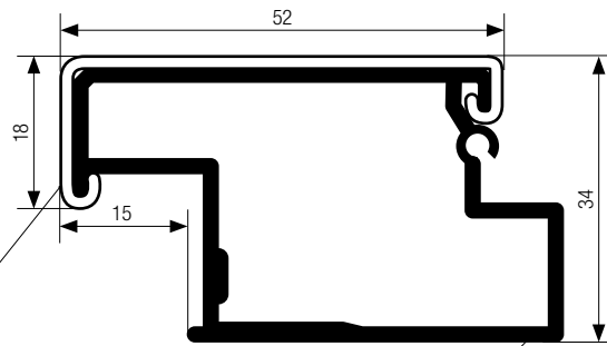
Griffleiste überlappend (Deckel) color-line / decor-line Griffleiste (Unterteil) color-line / decor-line (Alu)
