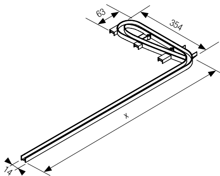
Führungsschnecke links und rechts : x = 400 / 500 / 600 mm Fassungsvermögen 600 mm
