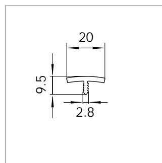
Mat.-Nr. 1718082 RAU-PVC 9608
