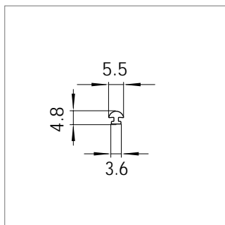
Mat.-Nr. 1626908 RAU-PVC 1309
