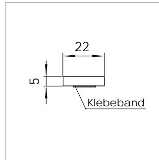
Mat.-Nr. 1630108 RAU-PVC 8200
