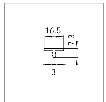
Mat.-Nr. 1715450 RAU-PVC 9600
