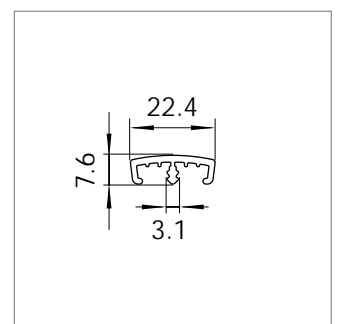
Mat.-Nr. 1712122* RAU-PP 1381
