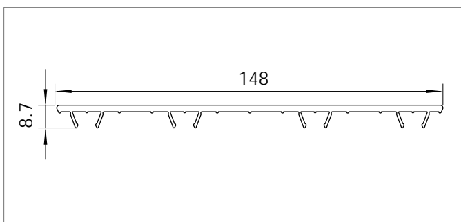
Mat.-Nr. 1628412 RAU-PVC 1309
