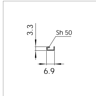
Mat.-Nr. 1624356 RAU-PVC 1107/5005
