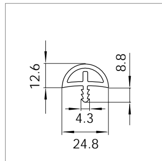
Mat.-Nr. 1712112 RAU-PVC 9008
