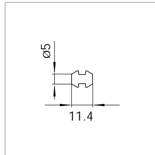
Mat.-Nr. 1956855 RAU-ABS 144
