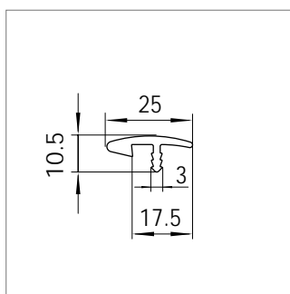
Mat.-Nr. 1713620 RAU-PVC 9600
