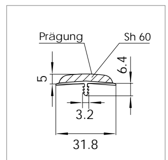
Prägung 237
