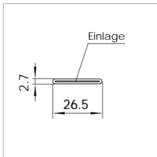
Mat.-Nr. 1308002 RAU-PVC 8200
