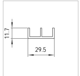
Mat.-Nr. 1625678* RAU-PVC 1309
