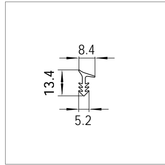
Mat.-Nr. 1956096 RAU-SRT 522
