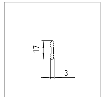
Mat.-Nr. 1622171 RAU-PVC 1200
