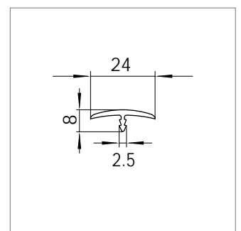
Mat.-Nr. 1718460 RAU-PVC 9600
