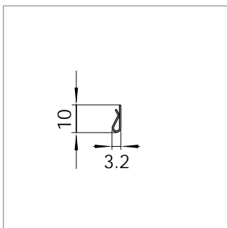
Mat.-Nr. 1739220 RAU-PVC 1203
