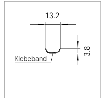
Mat.-Nr. 1604607 RAU-PE 759
