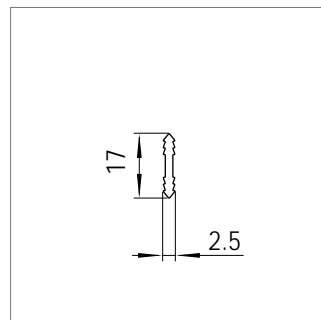
Mat.-Nr. 1634631 RAU-PVC 1200
