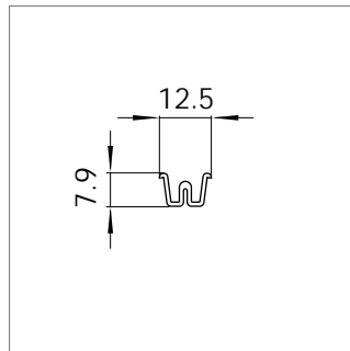
Mat.-Nr. 1770599 RAU-ABS 144
