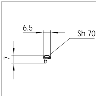
Mat.-Nr. 1619013 RAU-PVC 1134/7008
