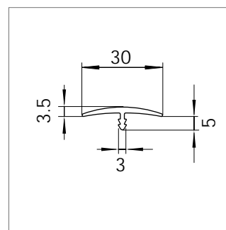
Mat.-Nr. 1718480 RAU-PVC 9600
