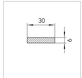
Mat.-Nr. 1302980 RAU-PVC 1309
