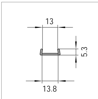
Mat.-Nr. 1752491 RAU-PVC 9400
