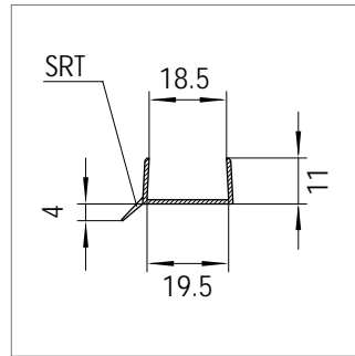
Mat.-Nr. 1609252 RAU-PVC 1299/8058
