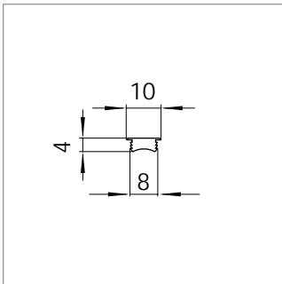
Mat.-Nr. 1607473 RAU-PVC 1103
