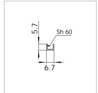
Mat.-Nr. 1626233 RAU-PVC 1107/6005
