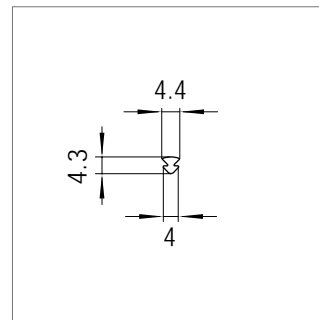
Mat.-Nr. 1609473 RAU-PVC 9008
