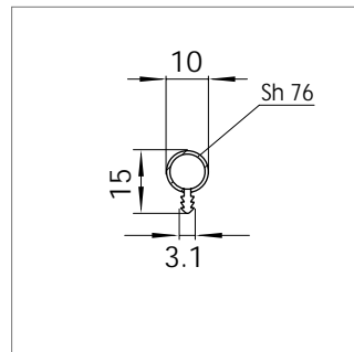
Mat.-Nr. 1635880 RAU-PVC 1200/7600
