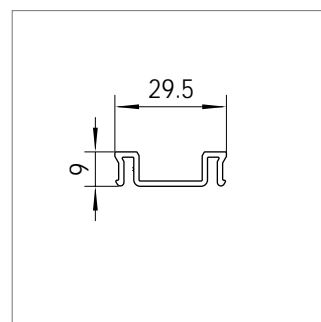
Mat.-Nr. 1616048 RAU-PE 130
