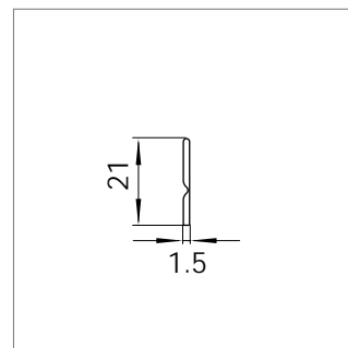
Mat.-Nr. 1403790* RAU-PP 236
