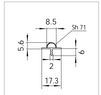
Mat.-Nr. 1608562 RAU-PVC 1203/7158
