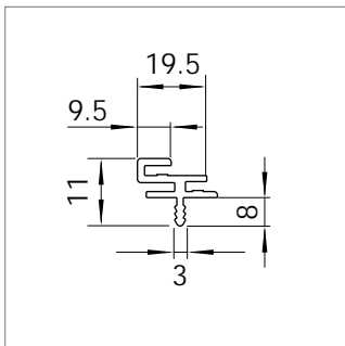
Mat.-Nr. 1625826* RAU-ABS 144
