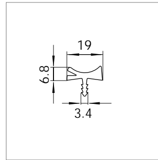
Mat.-Nr. 1712013* RAU-PVC 9298
