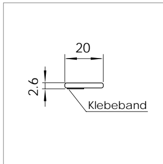
Mat.-Nr. 1956575* RAU-SB 159
