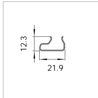
Mat.-Nr. 1626739 RAU-PVC 1309
