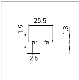
Mat.-Nr. 1956536* RAU-ABS 144
