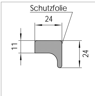
Mat.-Nr. 1636672 RAU-PVC 1203
