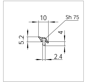
Mat.-Nr. 1712132 RAU-PVC 7500/1107
