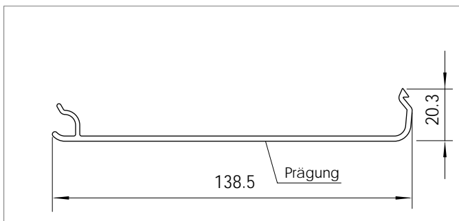
Mat.-Nr. 1634382 RAU-PVC 1103
