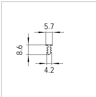
Mat.-Nr. 1718012 RAU-PVC 9600
