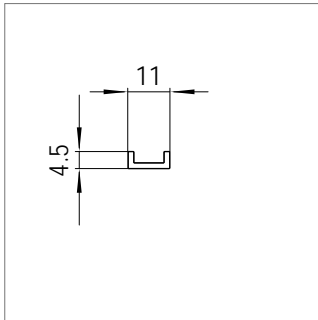
Mat.-Nr. 1625688* RAU-PVC 1309
