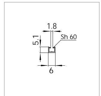
Mat.-Nr. 1620547 RAU-PVC 1107/6005
