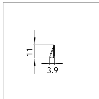
Mat.-Nr. 1956564 RAU-ABS 144
