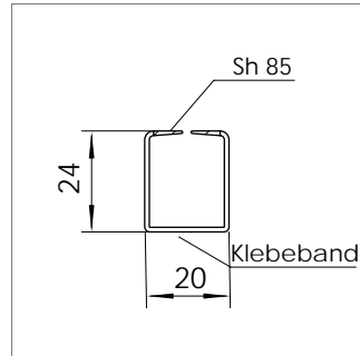
Mat.-Nr. 1637872 RAU-PVC 1520/8509
