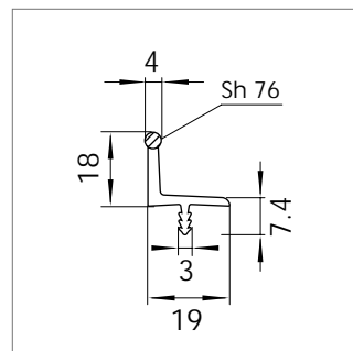
Mat.-Nr. 1603015 / 1603632 RAU-PVC 1203/7000
