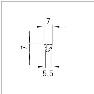
Mat.-Nr. 1607351 RAU-PVC 1200
