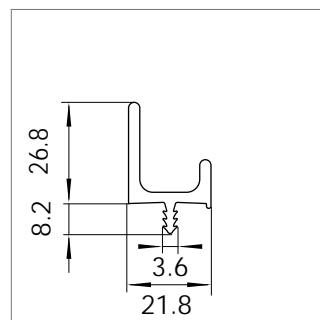
Mat.-Nr. 1616662 RAU-PVC 1309
