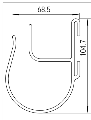
Mat.-Nr. 1956924 RAU-ABS 144
