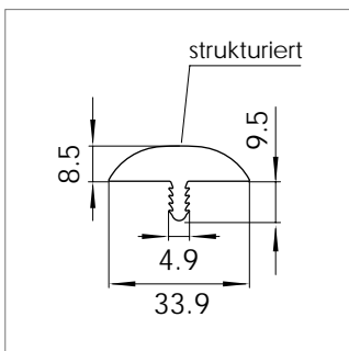
Mat.-Nr. 1712424 RAU-PVC 8508
