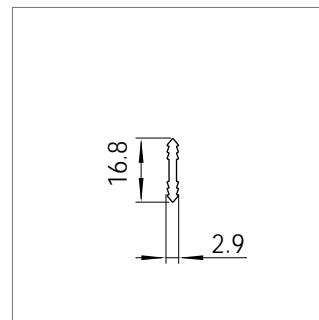
Mat.-Nr. 1605846 RAU-PVC 1200
