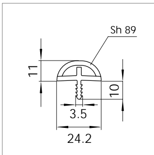
Mat.-Nr. 1718611* RAU-PVC 9608/8908
