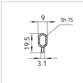
Mat.-Nr. 1623072 RAU-PVC 1203/7508
