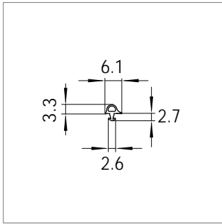
Mat.-Nr. 1856092/1834982 RAU-SIK 8760
