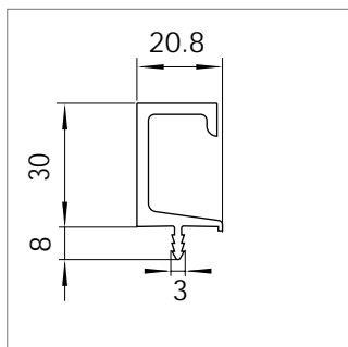
Mat.-Nr. 1637820 RAU-PVC 1309
