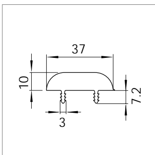
Mat.-Nr. 1718821 RAU-PVC 9008
