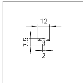
Mat.-Nr. 1956545 RAU-SRT 542
