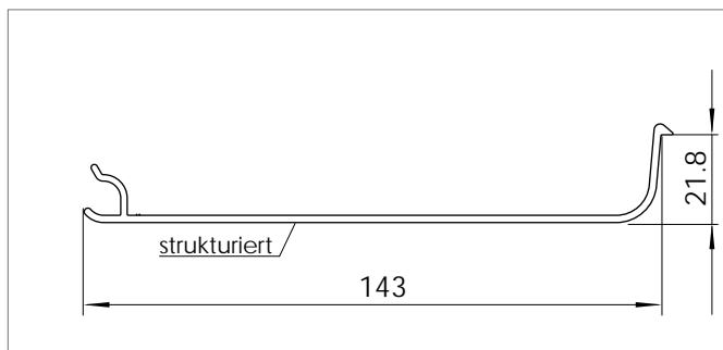
Mat.-Nr. 1615843 RAU-PVC 1309
