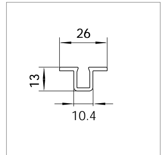
Mat.-Nr. 1625597 RAU-PVC 1309
