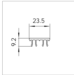
Mat.-Nr. 1608612 RAU-PVC 1309
