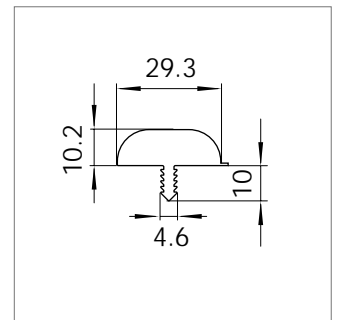
Mat.-Nr. 1711933 RAU-PVC 9008
