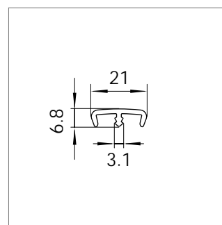
Mat.-Nr. 1712693 RAU-PP 1481
