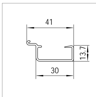
Mat.-Nr. 1621862 RAU-PVC 1309
