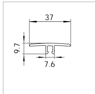
Mat.-Nr. 1628195 RAU-PVC 1309
