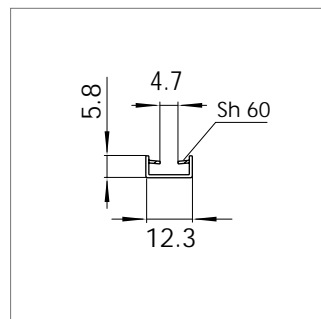
Mat.-Nr. 1628037 RAU-PVC 1107/6005
