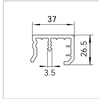
Mat.-Nr. 1626096 RAU-PP 136
