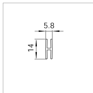
Mat.-Nr. 1619371 RAU-PVC 1309
