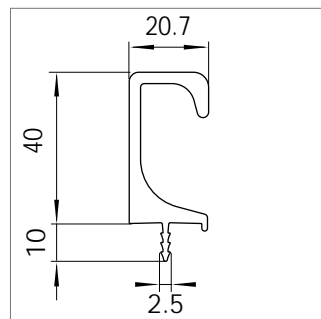
Mat.-Nr. 1632101 RAU-PVC 1309
