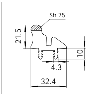
Mat.-Nr. 1601314* RAU-PVC 1103
