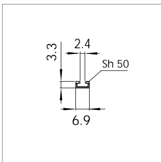
Mat.-Nr. 1628017 RAU-PVC 1107/5005
