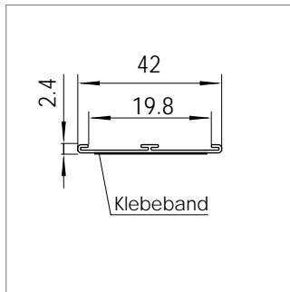
Mat.-Nr. 1719870 RAU-PVC 1299
