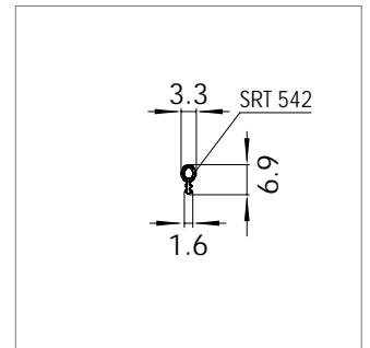
Mat.-Nr. 1621157 RAU-SRT 242/542
