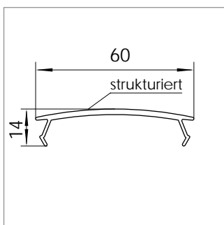
Mat.-Nr. 1612373 RAU-PVC 1309
