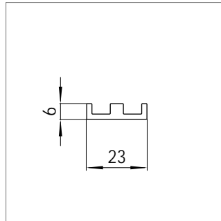
Mat.-Nr. 1622460 RAU-PVC 1200
