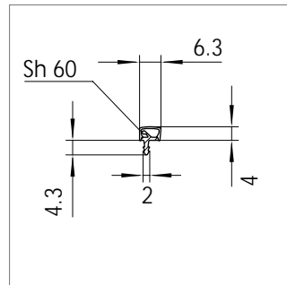
Mat.-Nr. 1604605 RAU-PVC 1134/6008
