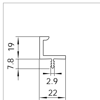
Mat.-Nr. 1633921 RAU-PVC 1299
