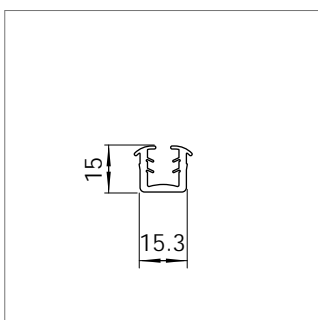
Mat.-Nr. 1637538* RAU-PVC 9058
