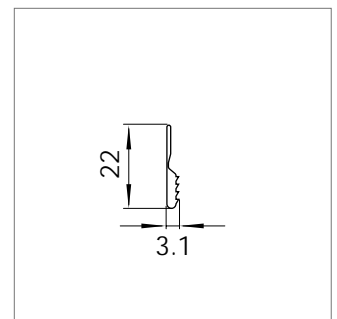
Mat.-Nr. 1400581* RAU-PVC 2504
