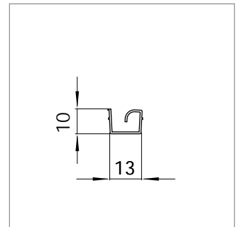
Mat.-Nr. 1625627* RAU-PVC 1107
