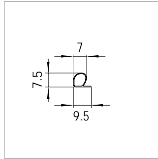
Mat.-Nr. 1858692 RAU-SIK 8158
