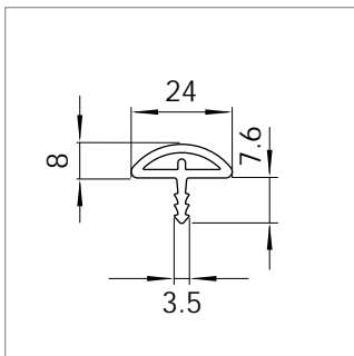
Mat.-Nr. 1625249 RAU-PVC 9505
