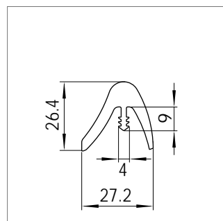
Mat.-Nr. 1712404 RAU-PVC 9458
