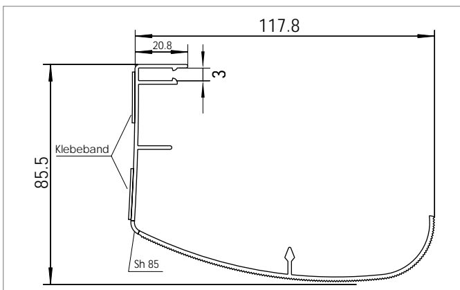
Mat.-Nr. 1733249* RAU-PVC 1389/8558
