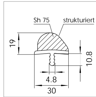
Mat.-Nr. 1712084* RAU-PVC 7558/9608
