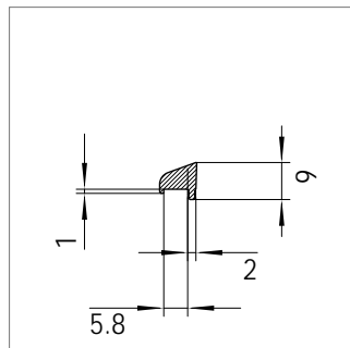
Mat.-Nr. 1618392 RAU-PVC 8500
