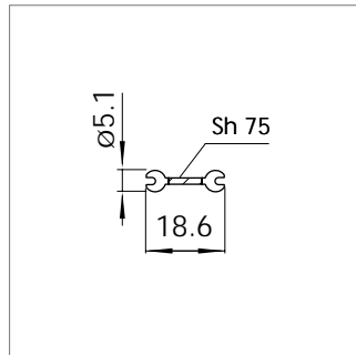
Mat.-Nr. 1625638 RAU-PVC 1309/7558
