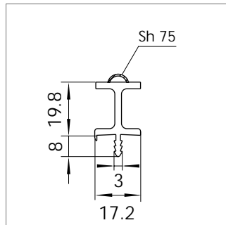
Mat.-Nr. 1632841 RAU-PVC 1299/7558
