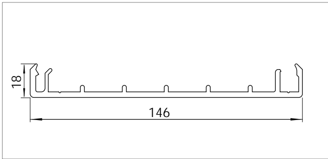
Mat.-Nr. 1725385* RAU-PVC 1309
