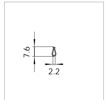
Mat.-Nr. 1739430 RAU-PVC 1200
