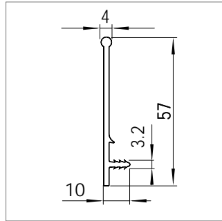
Mat.-Nr. 1718551 RAU-PVC 1309
