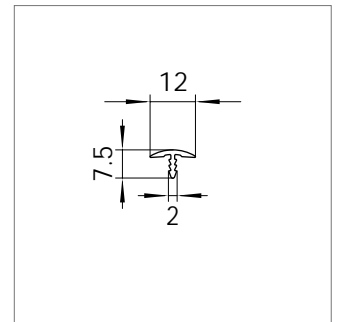
Mat.-Nr. 1715050 RAU-PVC 9600
